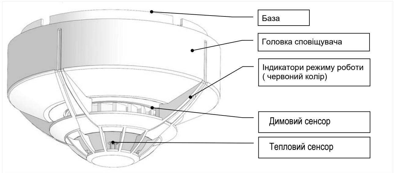
Рис 1. Зовнішній вигляд сповіщувача
