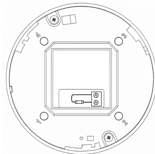
Рис 3. Встановлення обмежувального резистора
